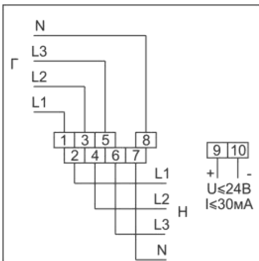
Рисунок Б.18 – Схема включения счетчиков в корпусах SP31 непосредственного включения
