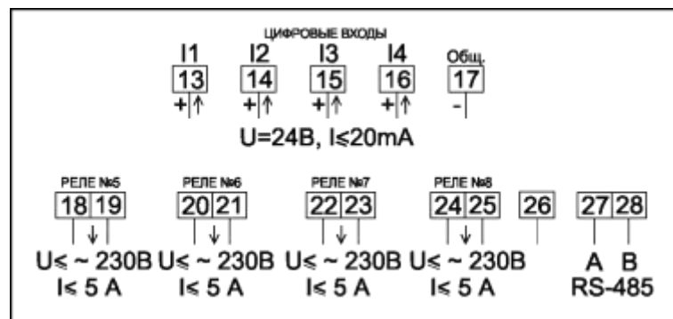
Рисунок Б.17 – Схема включения сигнальных цепей счетчиков в корпусах W32 с четырьмя дискретными выходами и четырьмя дискретными входами
