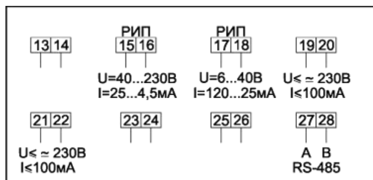
Рисунок Б.14 – Схема включения сигнальных цепей счетчиков в корпусах W30 2 с двумя дискретными выходами и резервным источником питания
