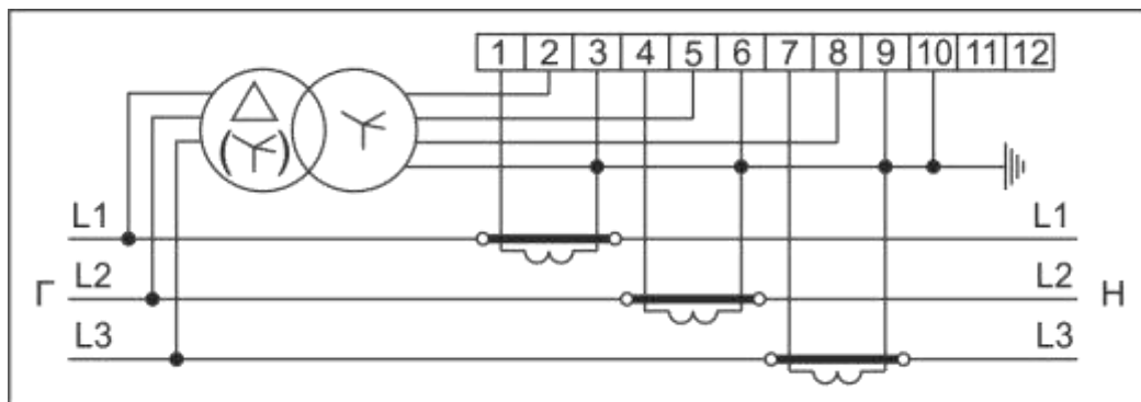
Рисунок Б.10 – Схема включения счетчиков в корпусах W32 через три трансформатора напряжения и три трансформатора тока
