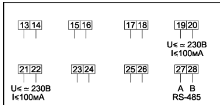
Рисунок Б.13 – Схема включения сигнальных цепей счетчиков в корпусах W32 с двумя дискретными выходами
