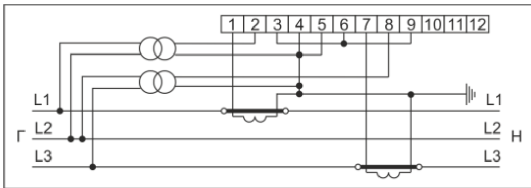
Рисунок Б.12– Схема включения счетчиков в корпусах W32 через два трансформатора напряжения и два трансформатора тока
