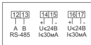
Рисунок Б.7 – Схема включения сигнальных цепей счетчиков в корпусах W31 и D33 со встроенным модулем интерфейса RS485 с двумя дискретными выходами
