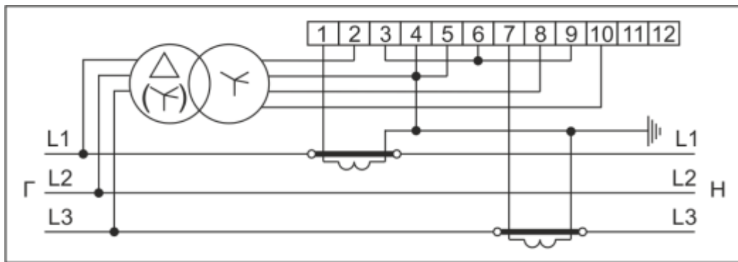
Рисунок Б.11 – Схема включения счетчиков в корпусах W32 через три трансформатора напряжения и два трансформатора тока
