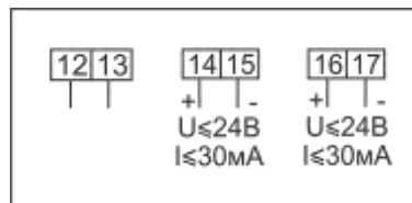
Рисунок Б.6 – Схема включения сигнальных цепей счетчиков в корпусах W31 и D33 с двумя дискретными выходами
