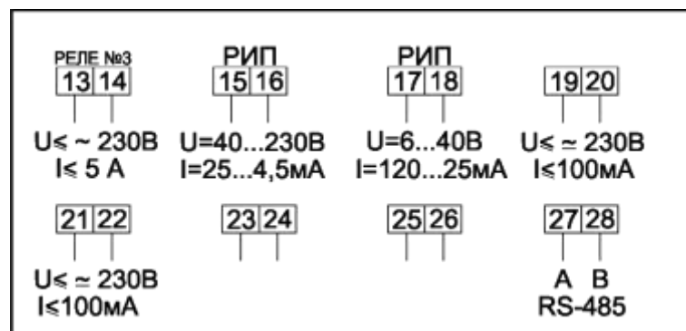
Рисунок Б.16 – Схема включения сигнальных цепей счетчиков в корпусах W32 с тремя дискретными выходами и резервным источником питания
