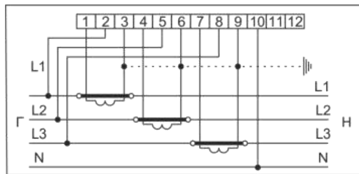
Рисунок Б.9 – Схема включения счетчиков в корпусах W32 через три трансформатора тока
