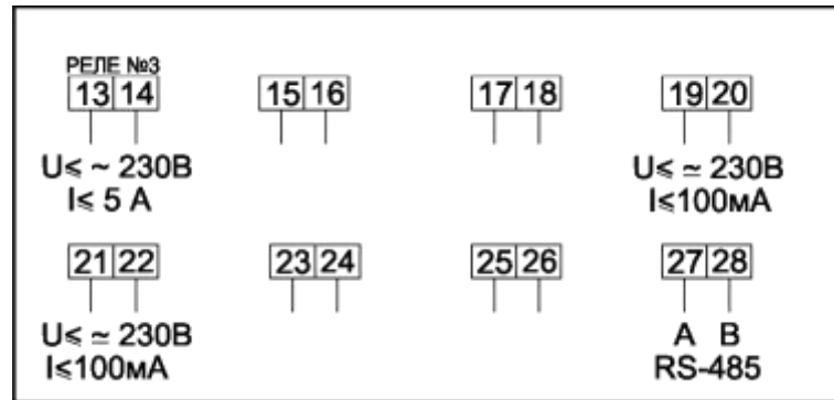
Рисунок Б.15 – Схема включения сигнальных цепей счетчиков в корпусах W32 с тремя дискретными выходами
